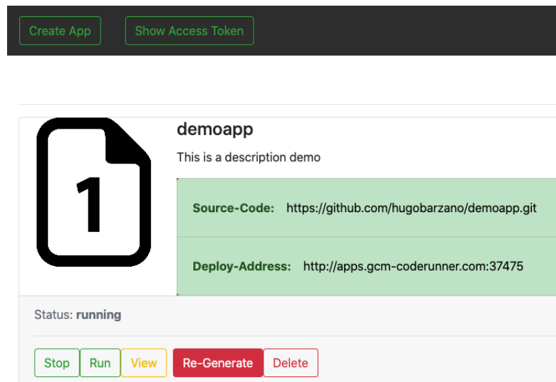
Figura 4.49: Re-Generación: Single-Page 0.0.2
