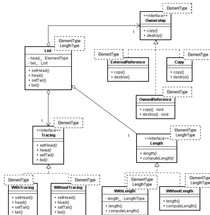
Figura 5.46. Diseño de una flexibilización del ejemplar basada en la composición y la herencia de clases.
