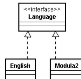
Figura 5.4. La especificación de cada diccionario implementará Language .
