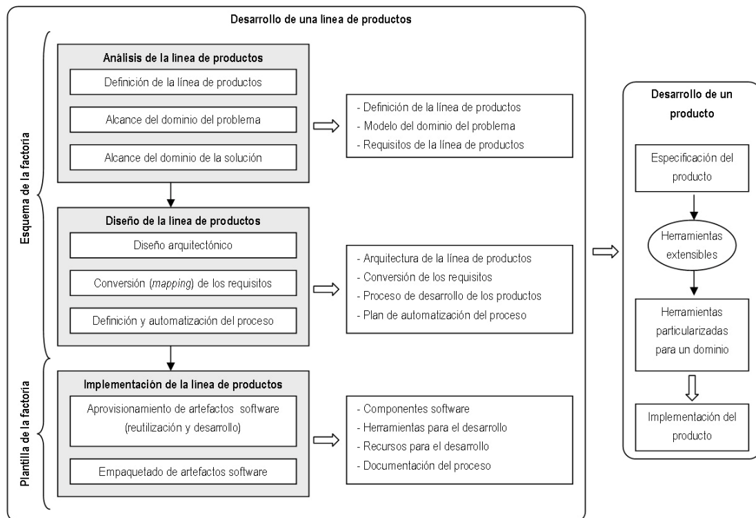
Figura 2.19. Principales procesos y productos de una factoría de software.
