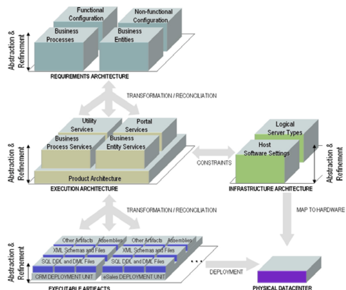
Figura 2.17. Representación mediante un grafo del esquema de una factoría de software propuesto por J. Greenfield [GS04]
