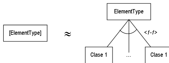
Figura 5.31. Equivalencia entre notaciones FODA.
